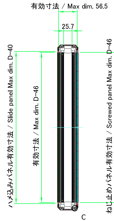
B-B ( 1 : 6 )
