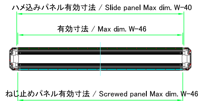
A-A ( 1 : 6 )
